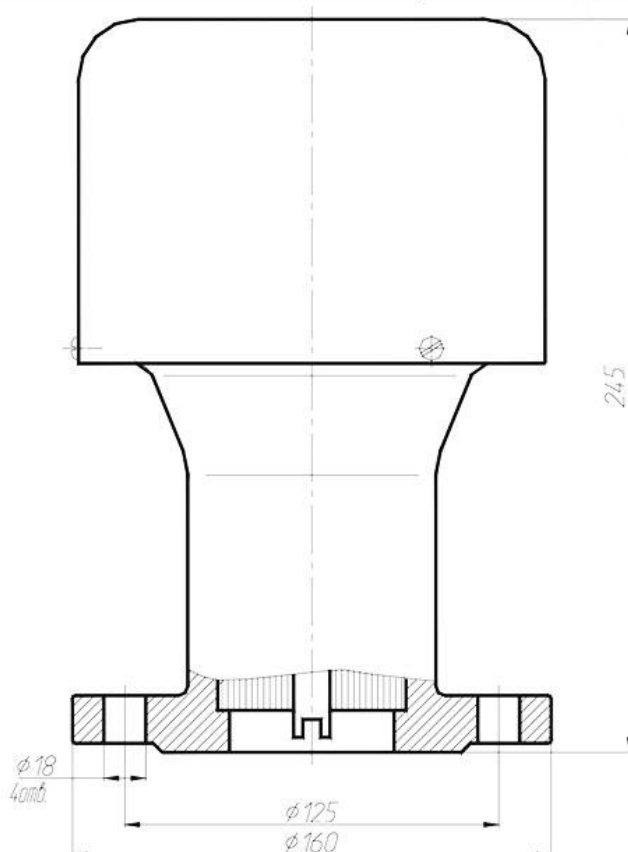
Общий вид клапана дыхательного механического КДМ-50М
