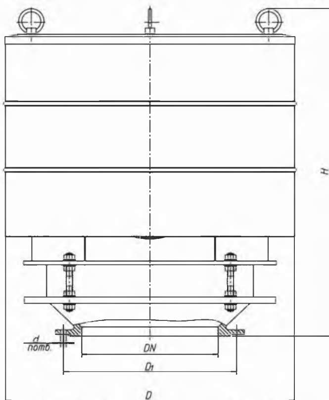
Общий вид клапана дыхательного КДС-1500К
