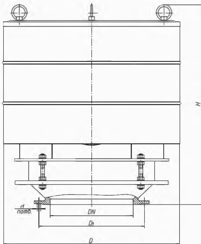
Общий вид клапана дыхательного КДС-3000К
