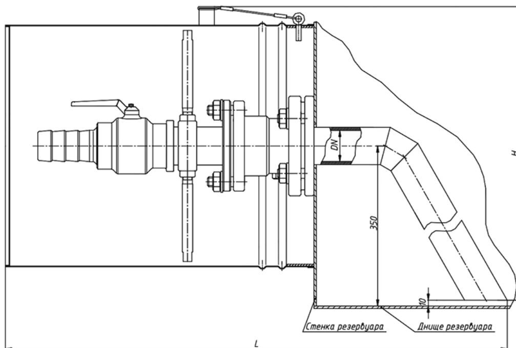
Общий вид крана сифонного КС
