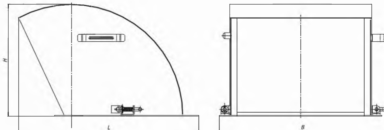
Общий вид патрубка вентиляционного периферийного ПВ п
