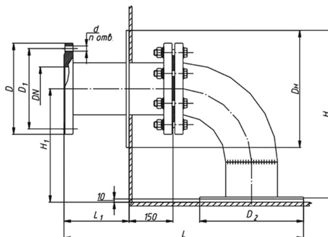
Общий вид патрубка зачистного ПЗ1
