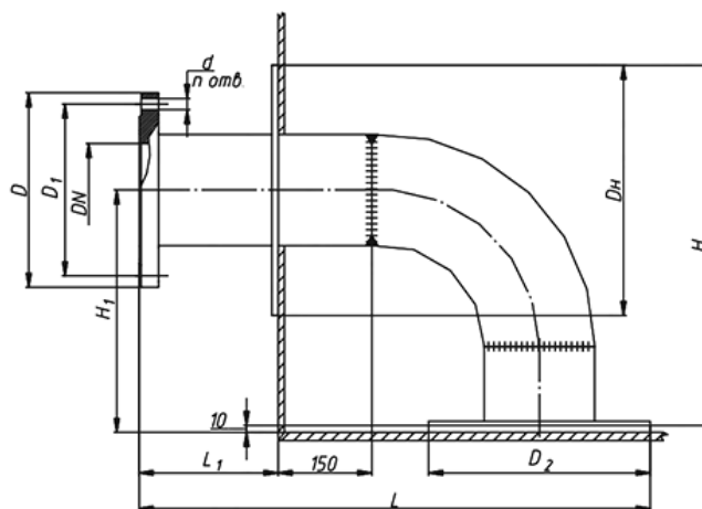
Общий вид патрубка зачистного ПЗ
