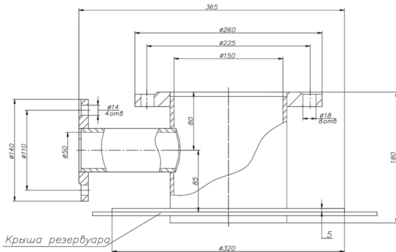
Общий вид патрубка замерного люка ПЗЛ-150
