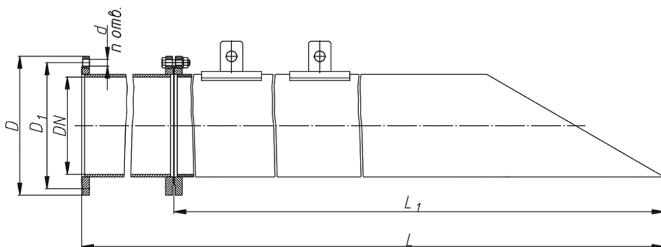
Общий вид трубы подъемной ТП
