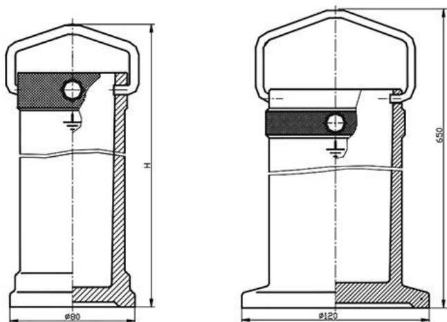
Общий вид ведерка замерного ВЗН-80, ВЗВ-80, ВЗВ-120
